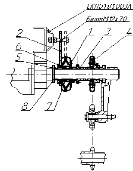
Рисунок 1 Разобщитель механизма привода
